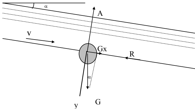
Hình 2.10. Sơ đồ lực tác động lên vật thể trôi
