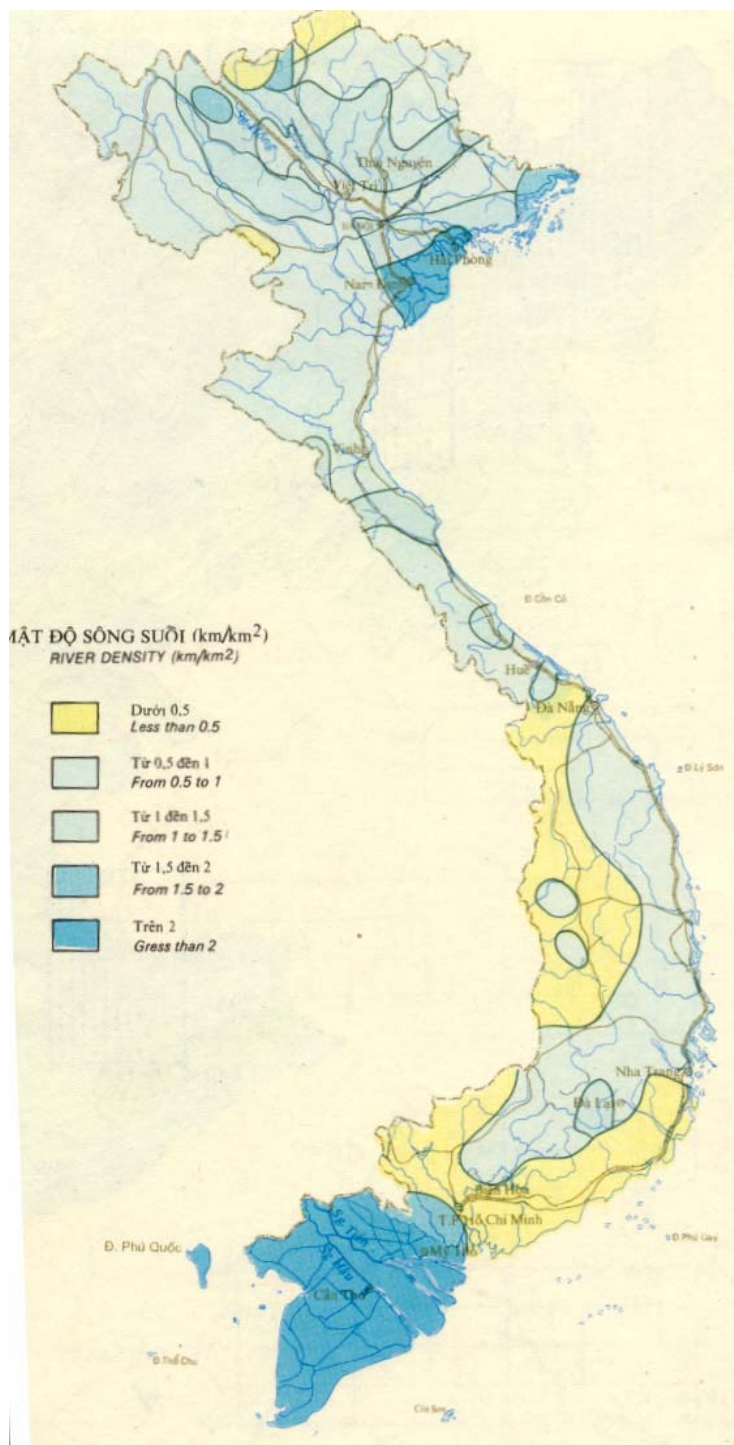
Hình 5.9. Mật độ sông suối
