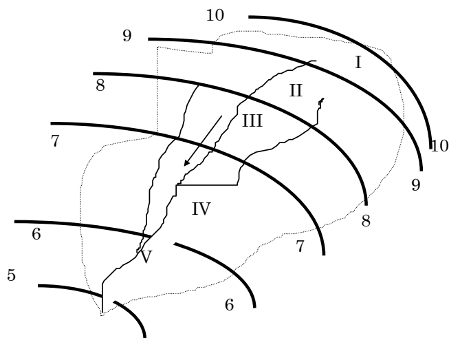
Hình 3.7 Sơ đồ xác định chuẩn dòng chảy năm theo bản đồ
