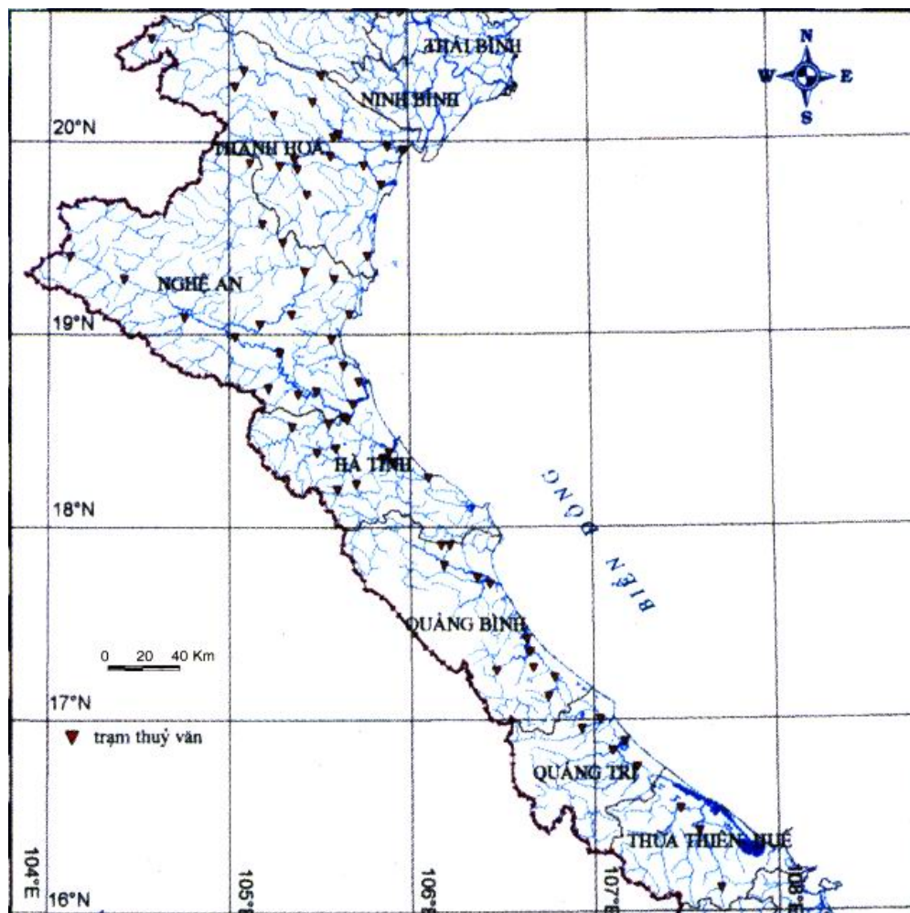
Hình 6.3 Sơ đồ hệ thống sông khu vực Bắc Trung Bộ
