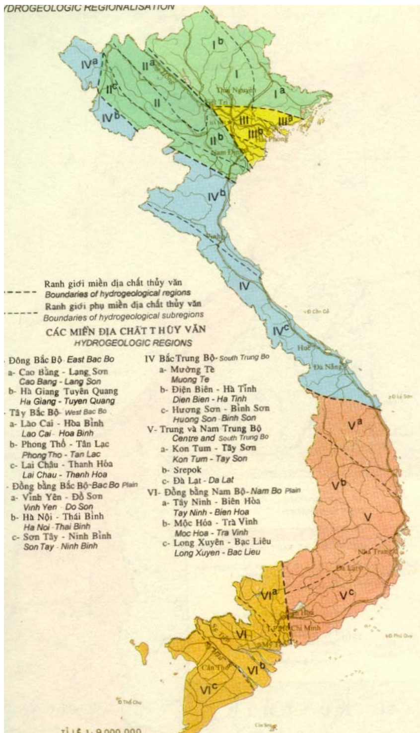
Hình 5.10. Bản đồ địa chất thủy văn
