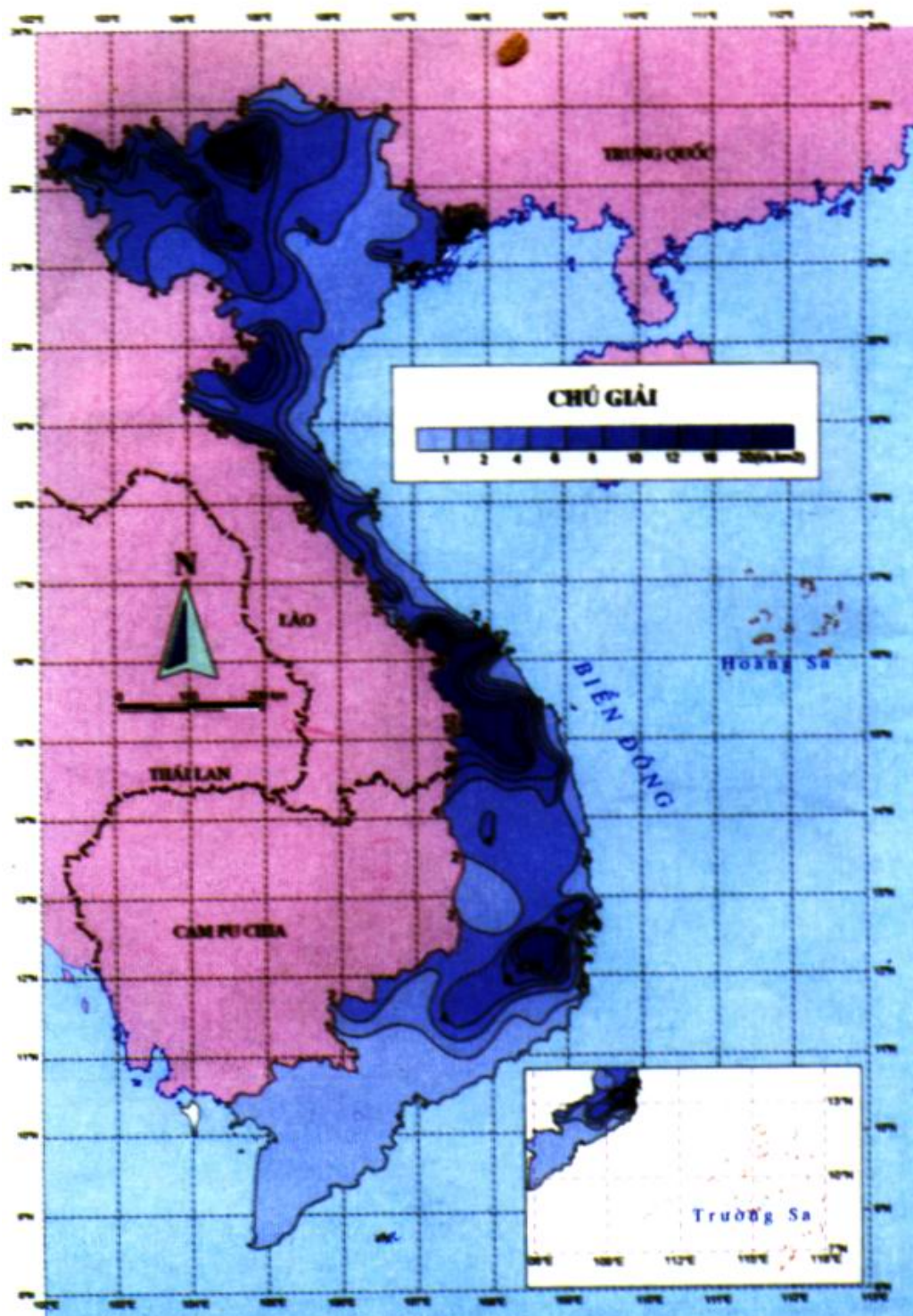
Hình 5.8. Bản đồ đẳng trị mô đun dòng chảy nhỏ nhất
