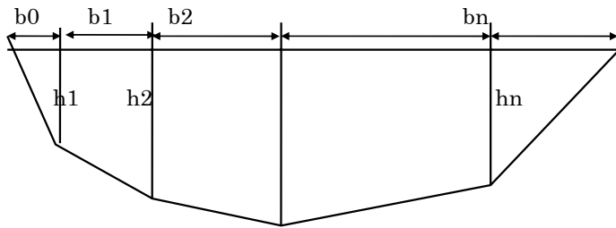
Hình 2.8. Sơ đồ tính diện tích mặt cắt ngang
