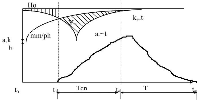
Hình 3.8. Sơ đồ khái quát quá trình mưa và quá trình dòng chảy
