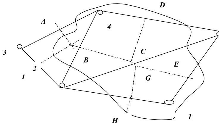
Hình 3.6. Phương pháp đường trung trực xác định mưa bình quân lưu vực
