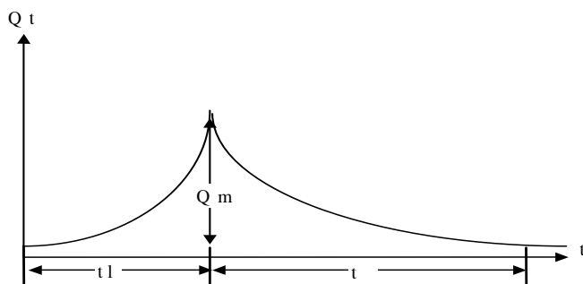
Hình 3.11 Mô hình hoá quá trình lũ parabol
