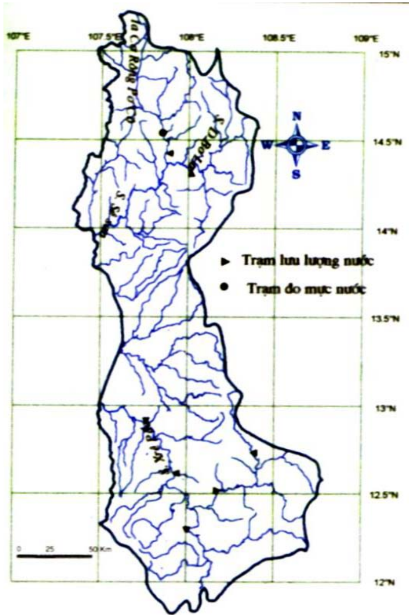
Hình 6.6. Sơ đồ lưới sông lưu vực sông SêSan và Xrê - pôc
