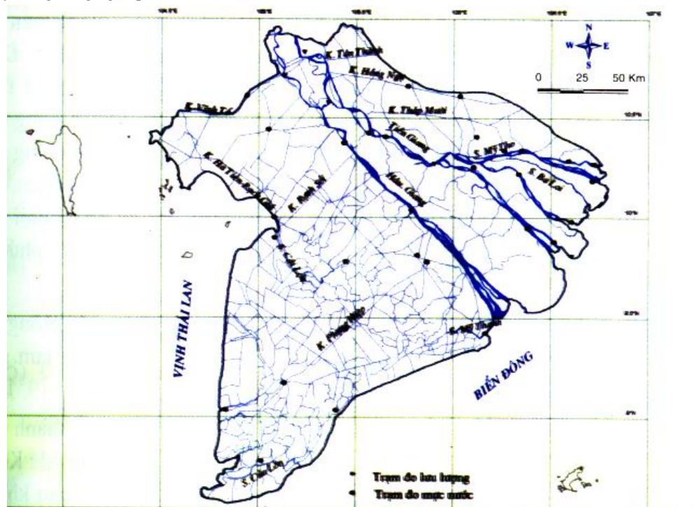
Hình 6.7. Sơ đồ lưới sông vùng đồng bằng sông Cửu Long
