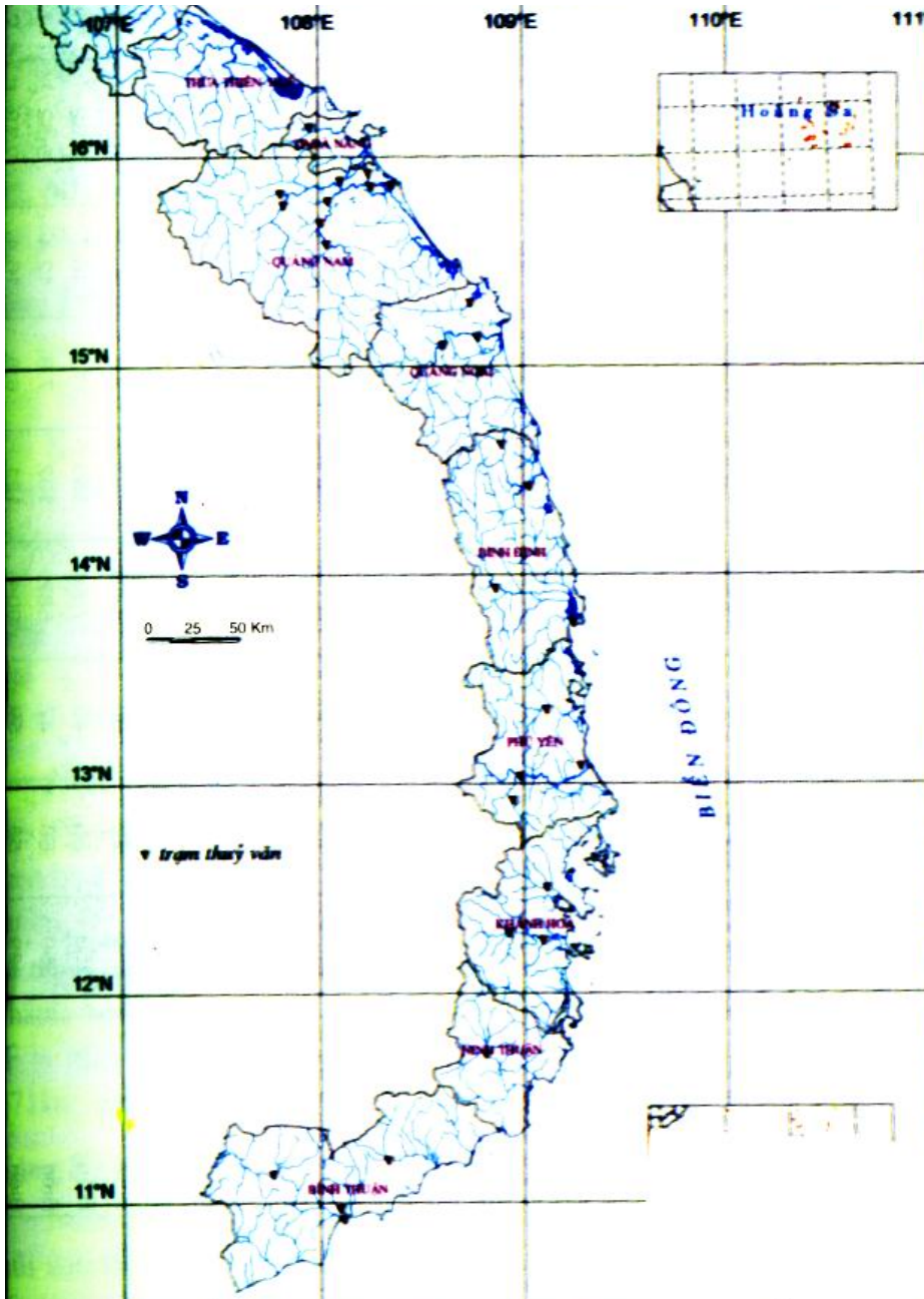
Hình 6.4. Sơ đồ hệ thống sông Nam Trung Bộ
