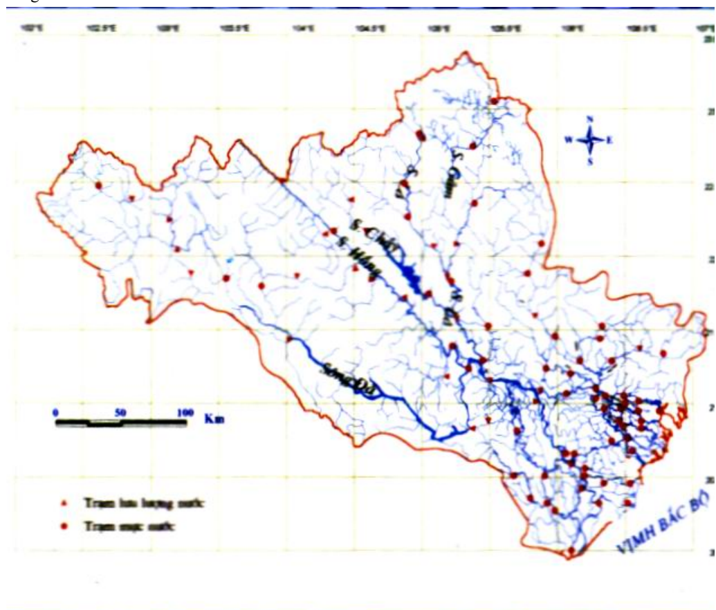
Hình 6.2. Sơ đồ lưới sông hệ thống Hồng - Thái Bình
