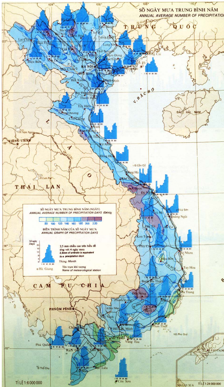
Hình 5.4. Bản đồ số ngày mưa trung bình năm
