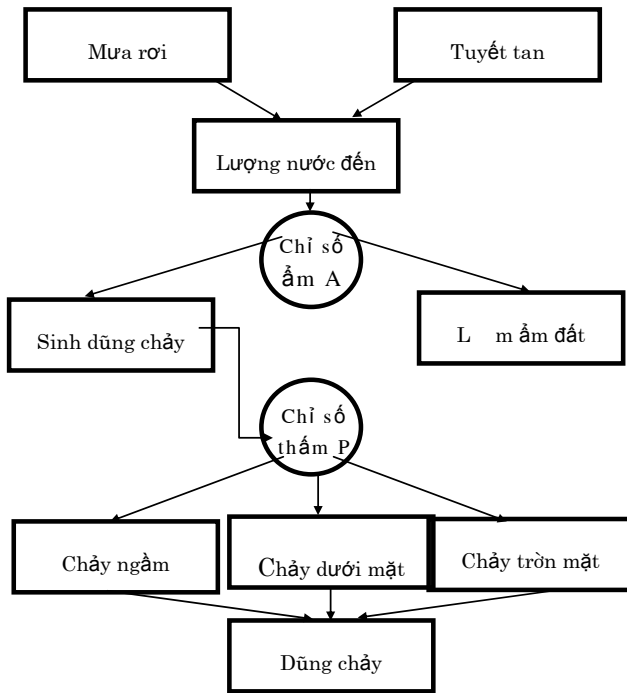
Hình 3.14. Sơ đồ mô hình lưu vực của mô hình SSARR \alpha = f_2(A)
