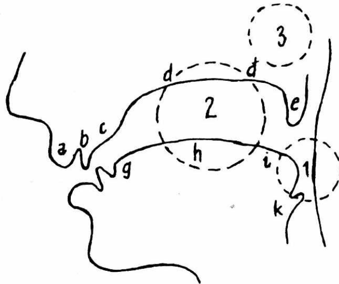
Hình 8. Các bộ phận của bộ máy phát âm và các khoang cộng hưởng trên thanh hầu: a) Môi; b) Răng; c) Lợi; d) Ngạc cứng; đ) Ngạc mềm; e) Lưỡi con; g) Đầu lưỡi; h) Mặt lưỡi trước; i) Mặt lưỡi sau; k) Nắp họng. 1. Khoang yết hầu; 2. Khoang miệng; 3. Khoang mũi.
